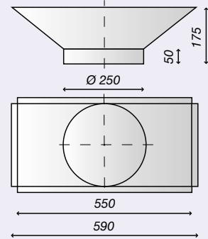
Filteraansluiting voor type C & D (2x)
