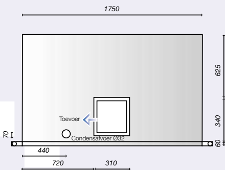
Achteraanzicht
