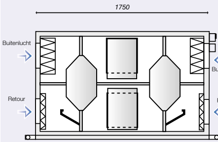
Vooraanzicht
