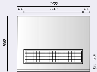
Linker/Rechter zijaanzicht
